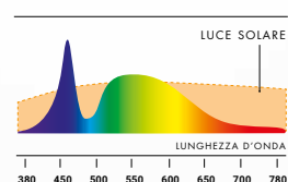
SPETTRO LAMPADINE A LED IN COMMERCIO
